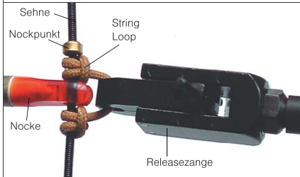
String Loop / Releasezange
