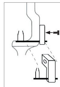
Beispiel : Anbringung der Pfeilauflage MUSTANG
